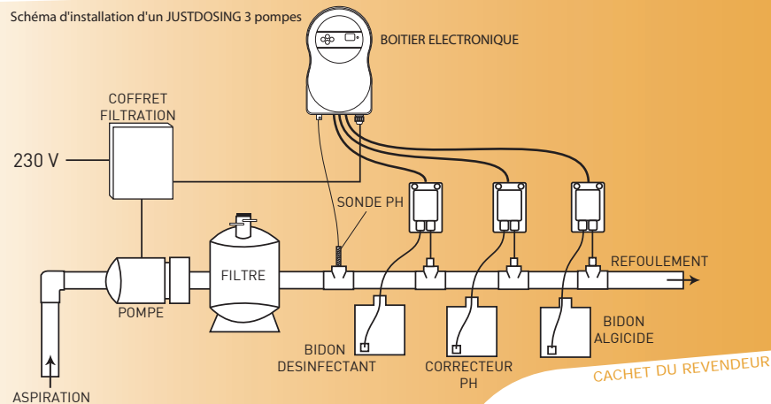
Schéma d'installation d'un JUSTDOSING 3 pompes
